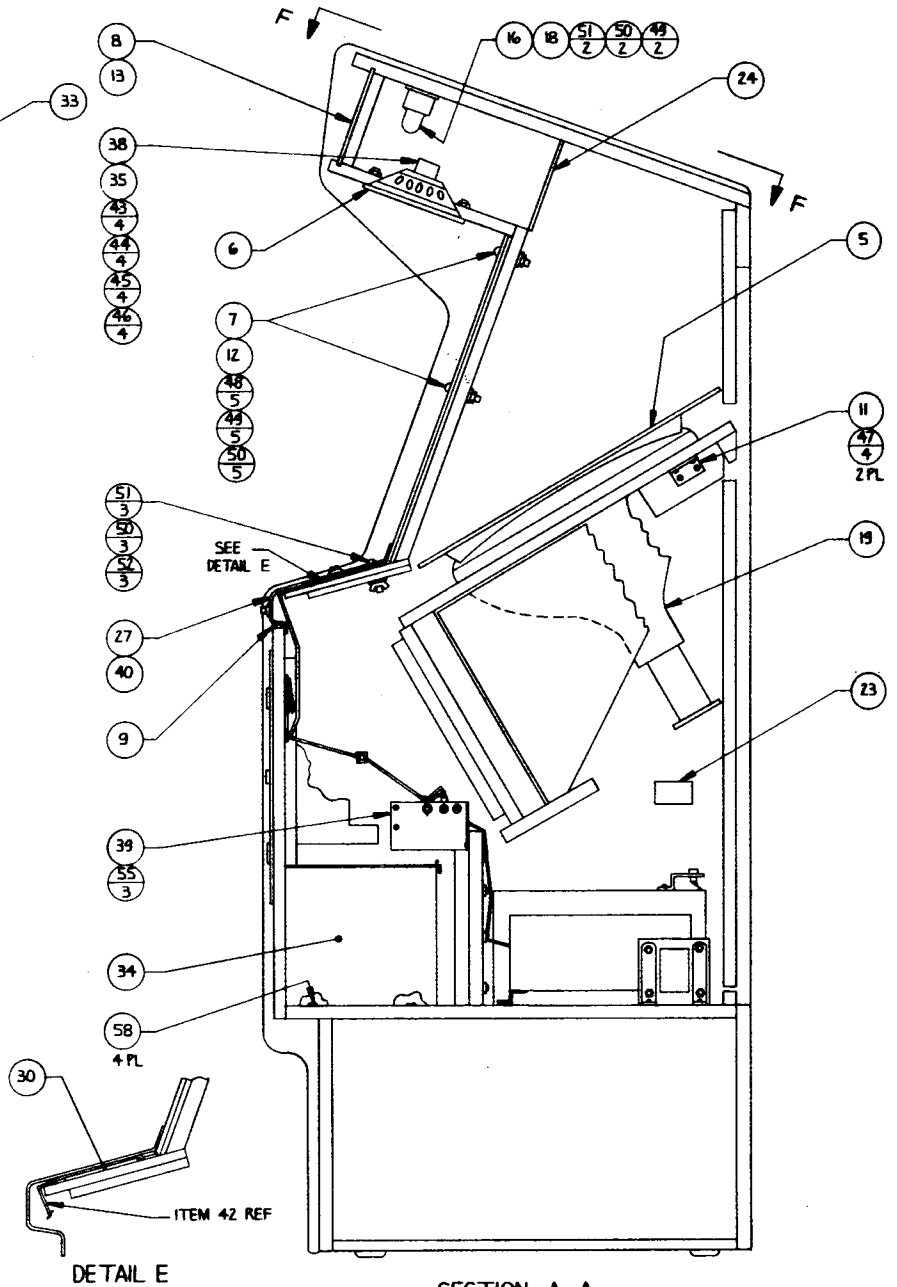
SECTION A-A
