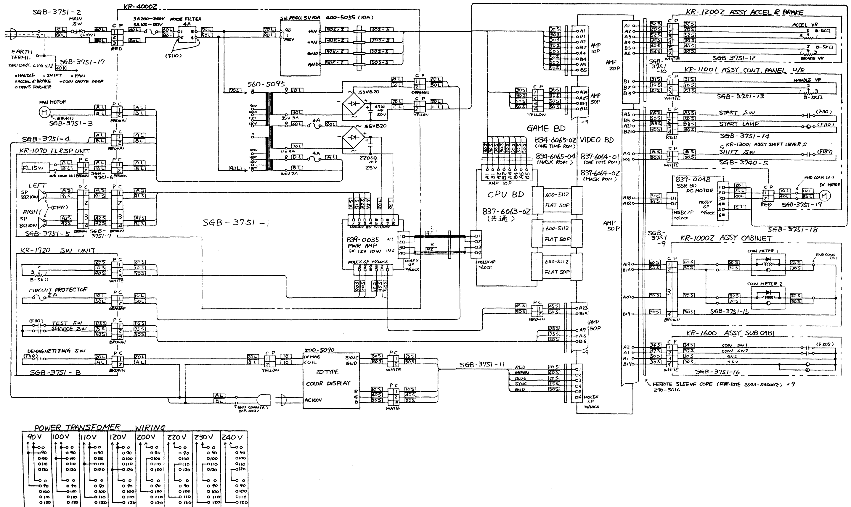
15. WIRING DIAGRAM
