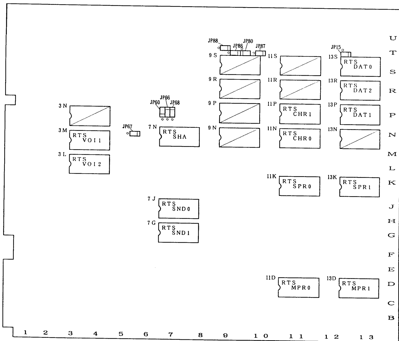
図3 (CPU-PCボード)
