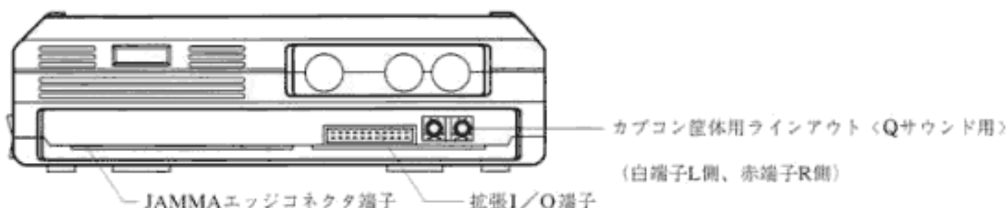
端子面
