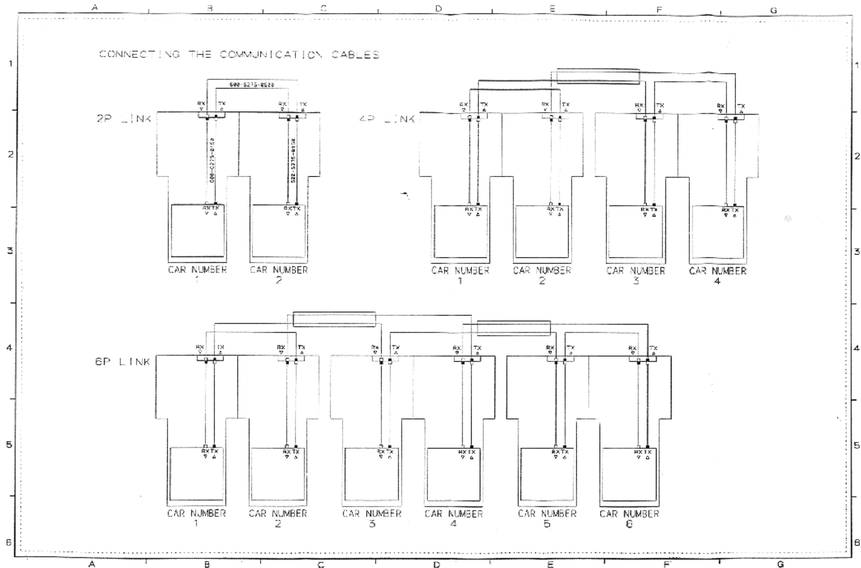
23. WIRING DIAGRAM (D-4/5)
